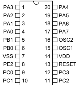
HT82K68E -20 SOP-A
