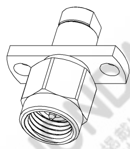
外観図 Appearance
