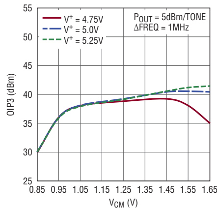
OIP3 at 380MHz vs V_{CM} Over V^+
