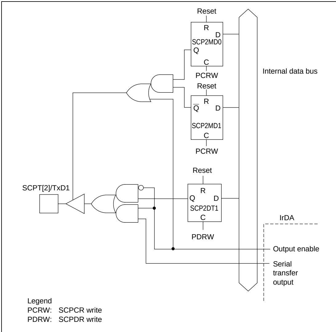
Figure 17.3 SCPT[2]/TxD1 Pin
