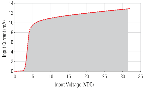
4-32 VDC Input
