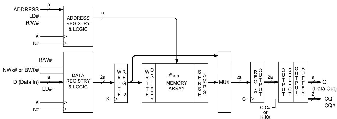
Figure 2: Functional Block Diagram 4 Meg x 8; 4 Meg x 9; 2 Meg x 18; 1 Meg x 36
