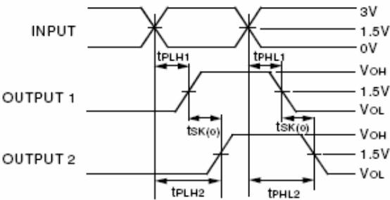
Output Skew - tSK(0)
