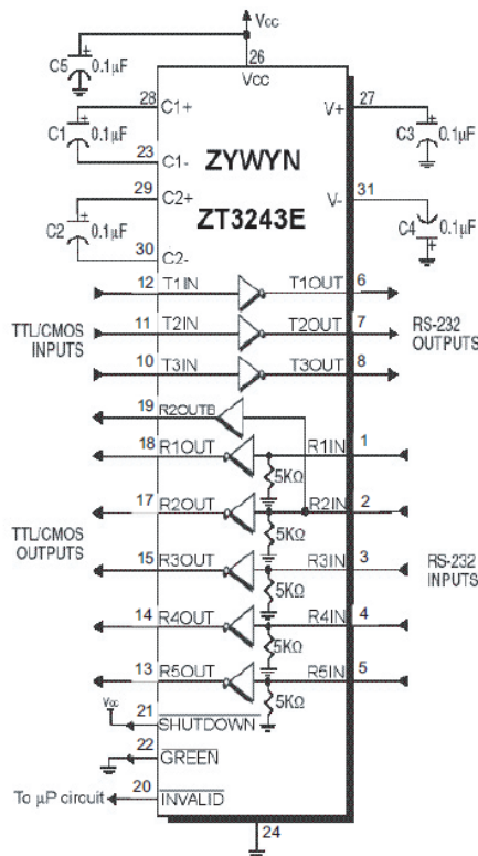
ZT3243E VQFN
