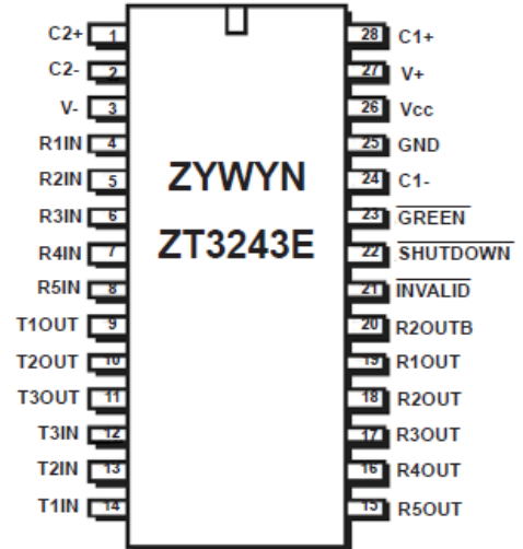
28-Pin SSOP/TSSOP/WSOIC
