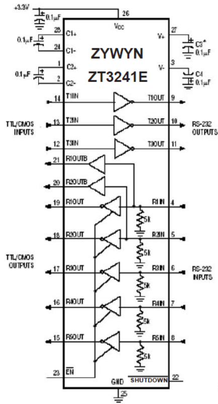
ZT3241E SSOP, wSOIC
