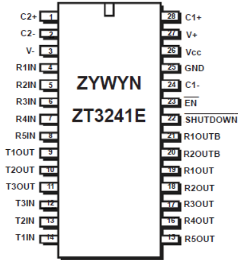
28-Pin SSOP/TSSOP/WSOIC
