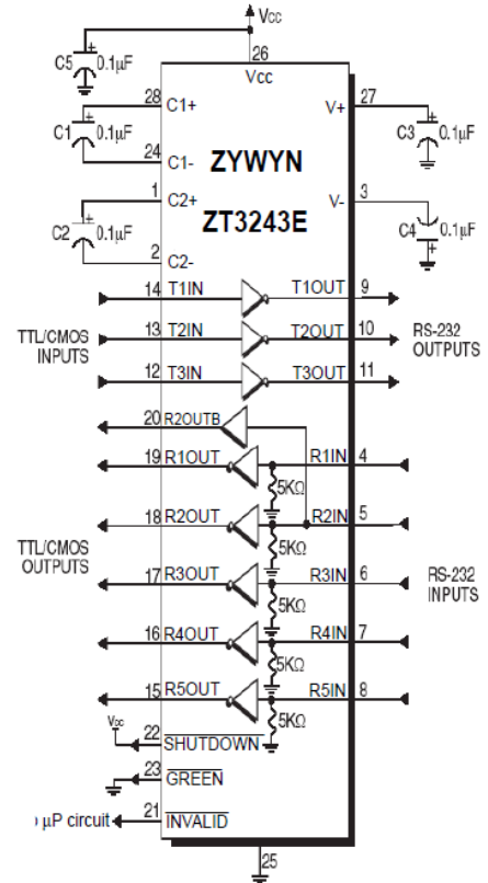
ZT3243E SSOP, wSOIC, TSSOP
