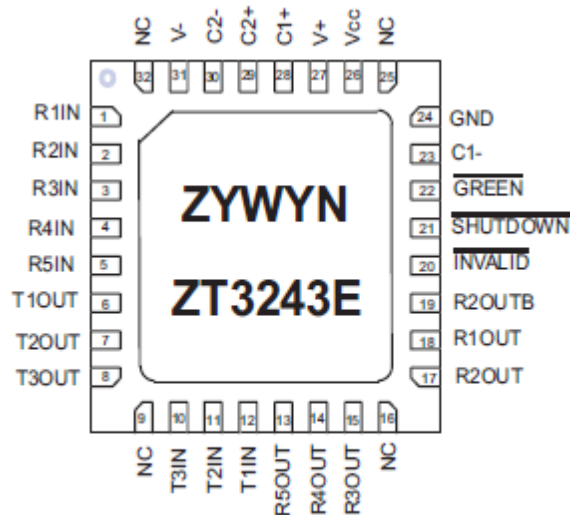
32-Pin VQFN
