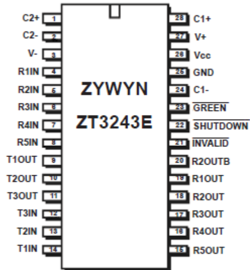
28-pin SSOP/TSSOP/WSOIC
