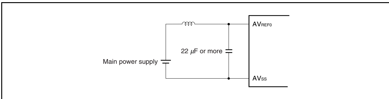
Figure 13-14. AV REF0 Pin Processing Example
