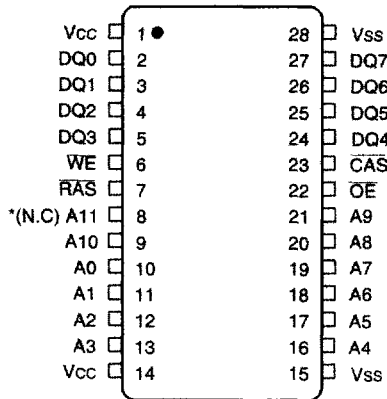
28Pin Plastic SOJ (300mil)
