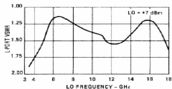
VSWR
