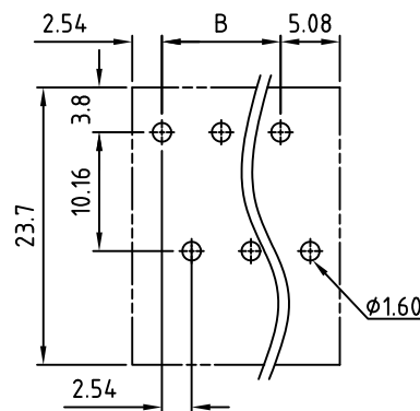
P.C.Board Layout
