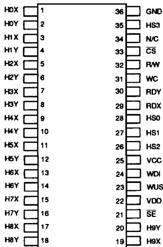
SSI 32R2101R 36-Lead, TTL Input 10-Channel SOM
