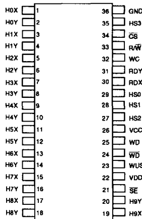
SSI 32R2100R - 36-Lead, 10-Channel SOM
