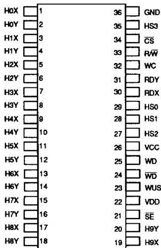
SSI 32R2100R 36-Lead, PECL Input 10-Channel SOM
