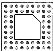
56 PINS PATTERN 0907
