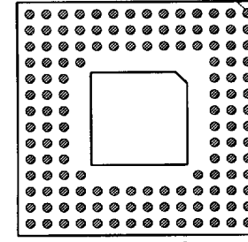
135 PINS PATTERN 1410
