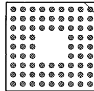
72 PINS PATTERN 0904
