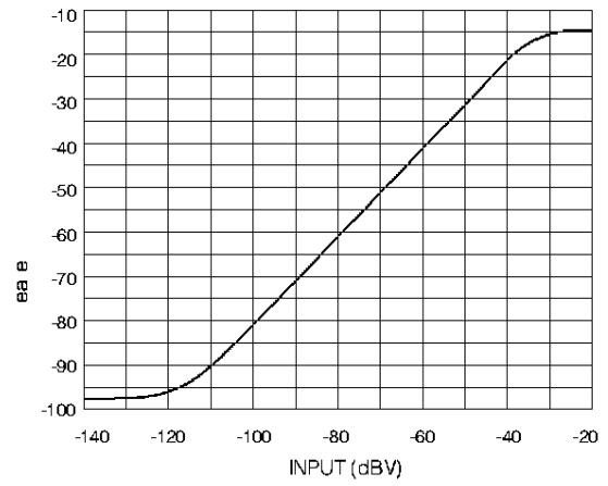
Fig. 6 Input vs Output (Telecoil)
