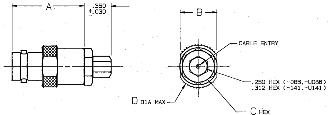
FIG 2 - 086 SHOWN
