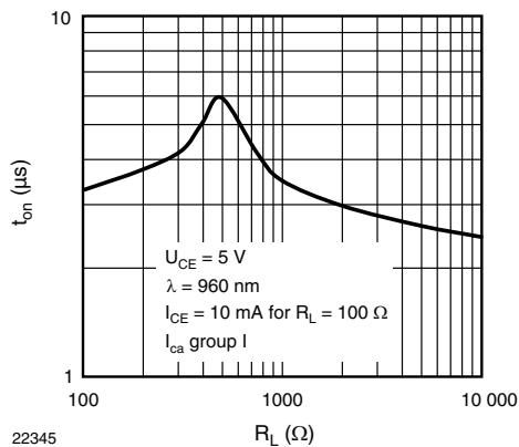
Fig. 2 - Turn-on Time
