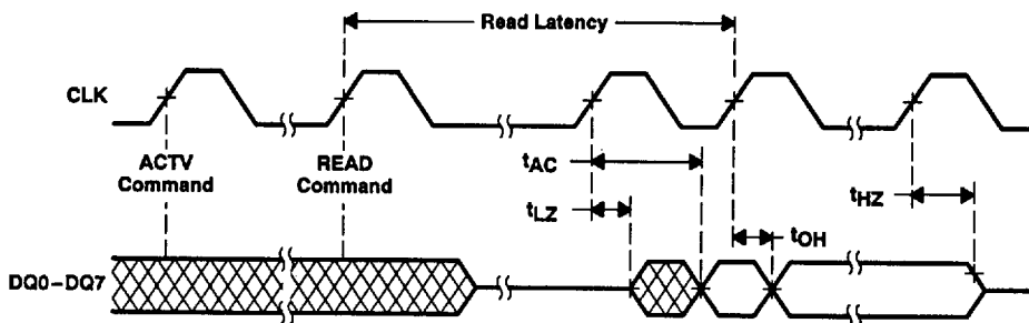
Figure 12. Output Parameters
