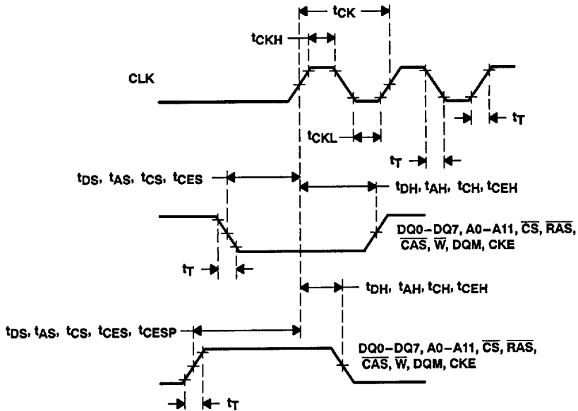
Figure 14. Input-Attribute Parameters
