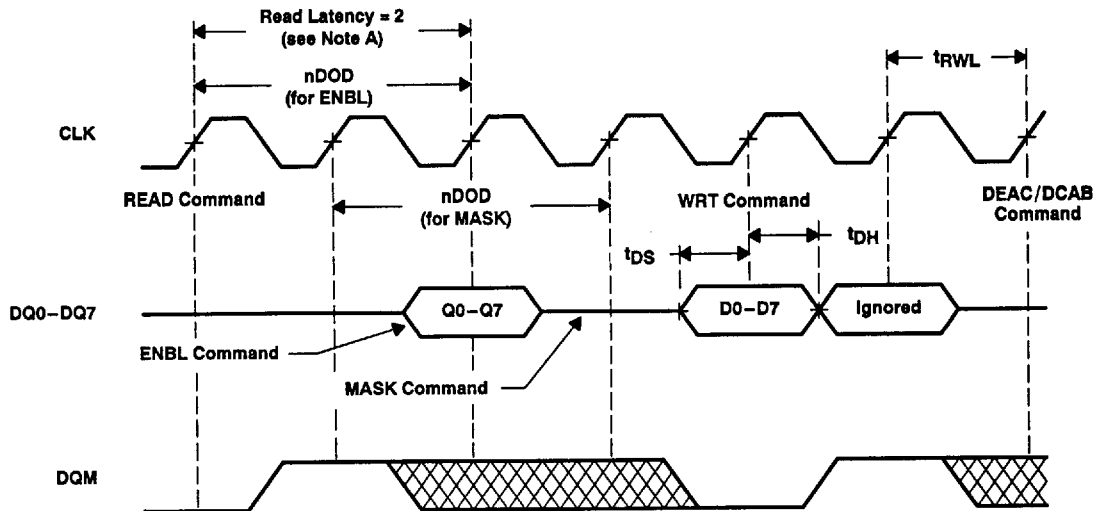
Figure 15. DQ Masking
