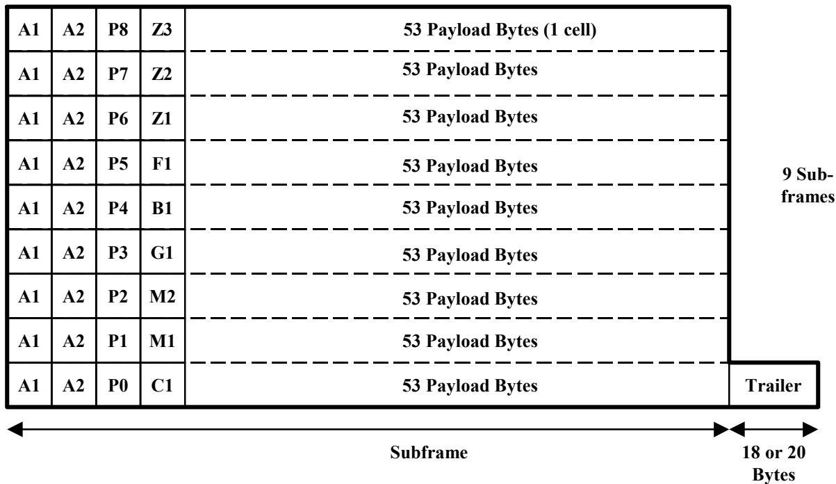
Figure 10-12. E3 PLCP Frame
