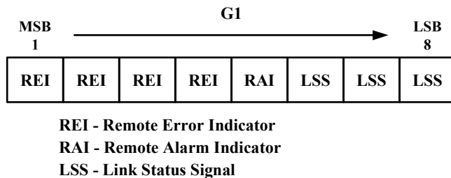
Figure 10-30. E3 PLCP G1 Byte Format
