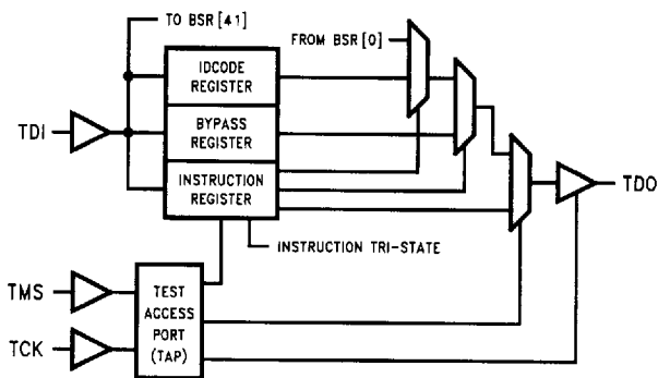
Tap Controller
