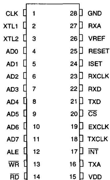
300-Mil 28-Pin DIP 73K224L-IP
