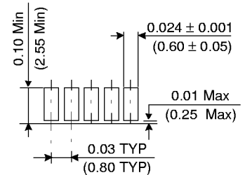
Detail Y
