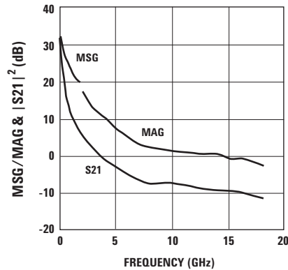
Figure 36. MSG/MAG & |S_{21}|^2 (dB) @ 3V, 200 mA.
