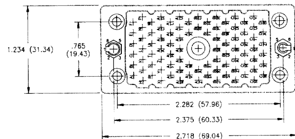
120 PIN RECEPTACLE
