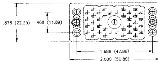
38 PIN RECEPTACLE
