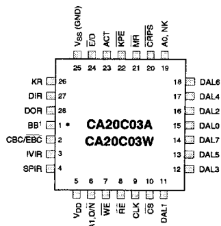
b) 28-pin PLCC
