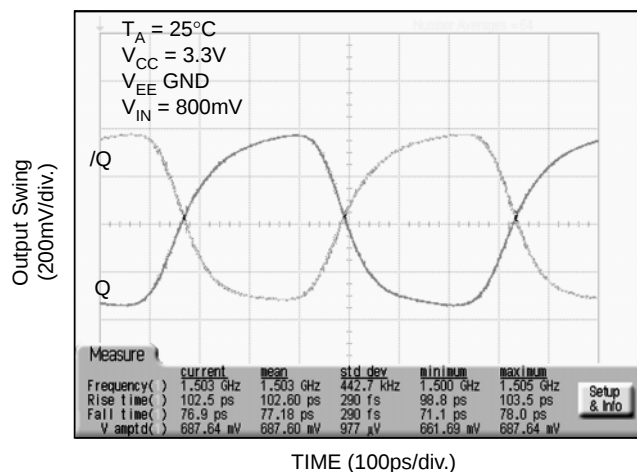
1.5GHz Output
