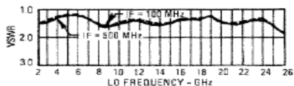
I-Port VSWR
