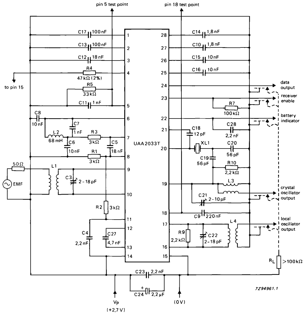
Fig. 3 Test circuit.
