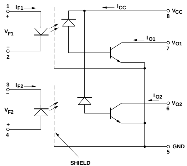
HCPL-253L/HCPL-053L
