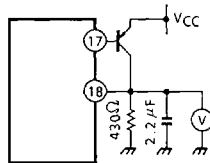
(10) V_{REG}
