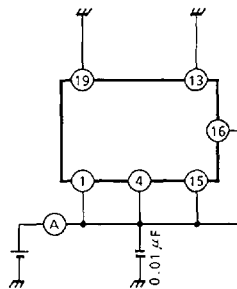
I_{CCO}
