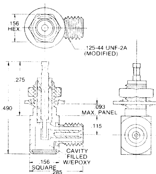
RIGHT ANGLE RECEPTACLE 141-0013-0001
