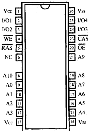
24(26) SOJ
