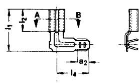
Schnitt A-B
