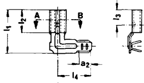
Schnitt A-B
