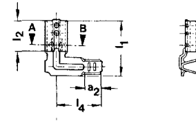
Schnitt A-B
