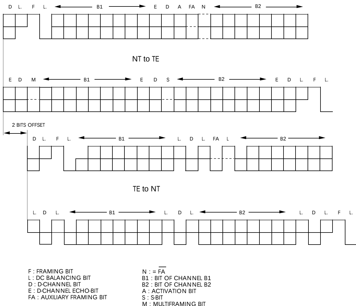
Fig. 20 : So-Frame Format
