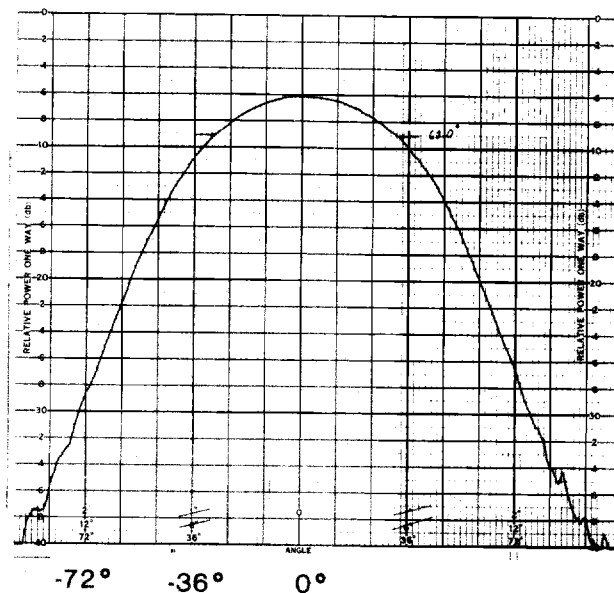
H-Plane — A-Band
