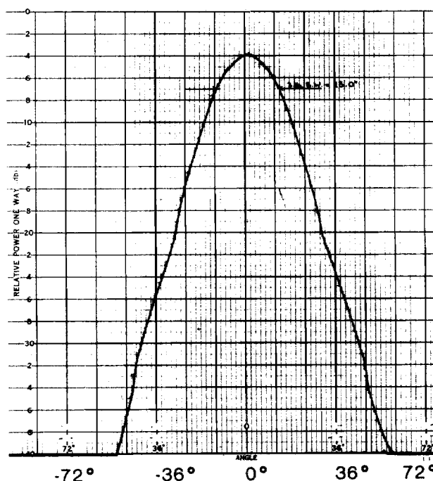
H-Plane — K-Band
