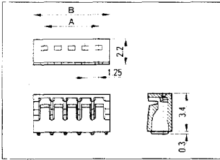
DIP CONNECTOR ディップコネクタ (1.25mmピッチ)
