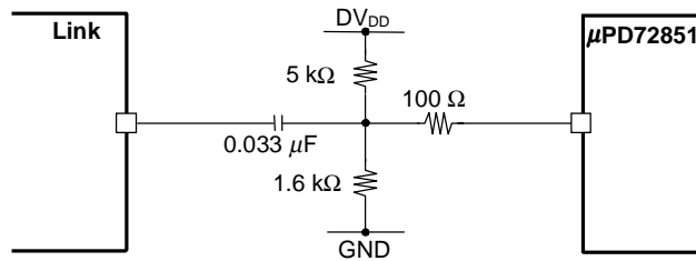
(d) LREQ Isolation Barrier Circuit
