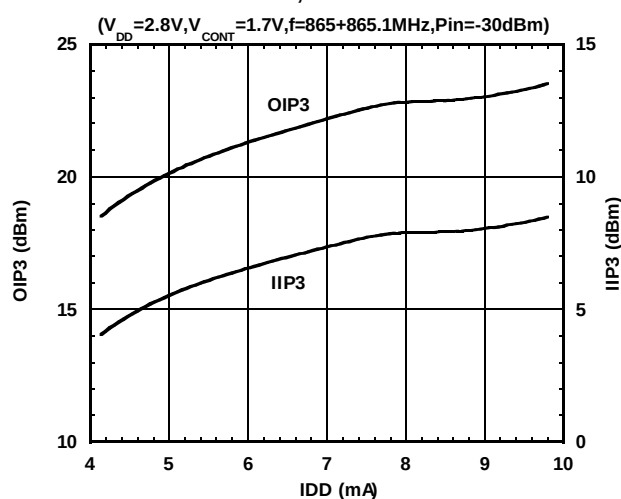
OIP3, IIP3 vs. IDD
