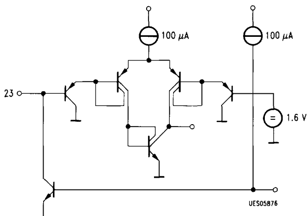
I²C Bus SDA (Pin 23)
