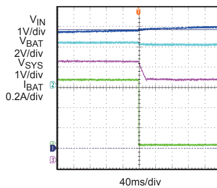
Input OVP
