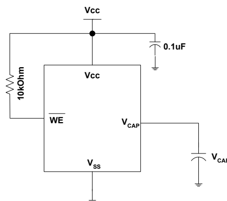
Figure 3. AutoStore Mode
