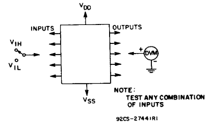
Fig. 14 - Input voltage.
