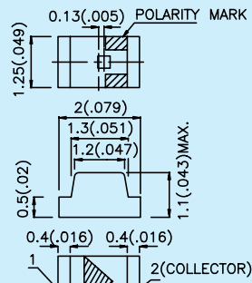
KP-2012P3 2.0mm x 1.25mm x 1.1mm (0805)
