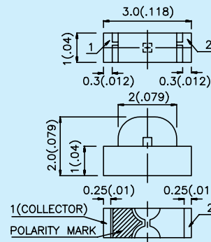
KPA-3010P3 3.0mm x 1.0mm x 2.0mm (1104)
