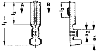
Schnitt A-B
