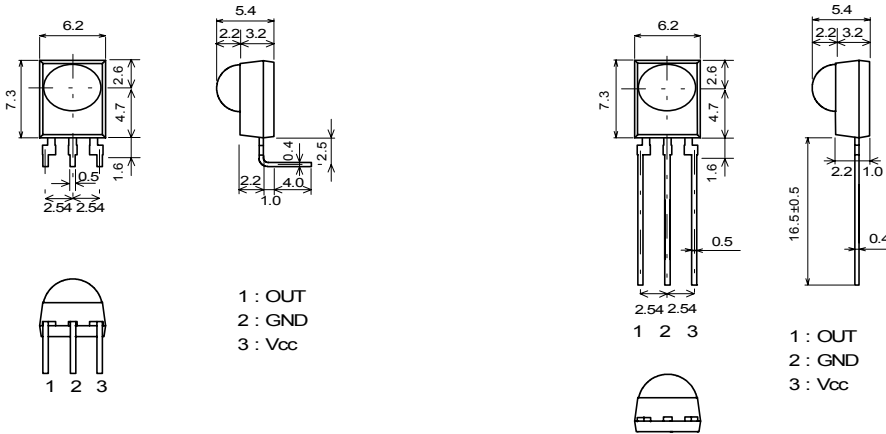
NJL71H000A UNIT:mm
