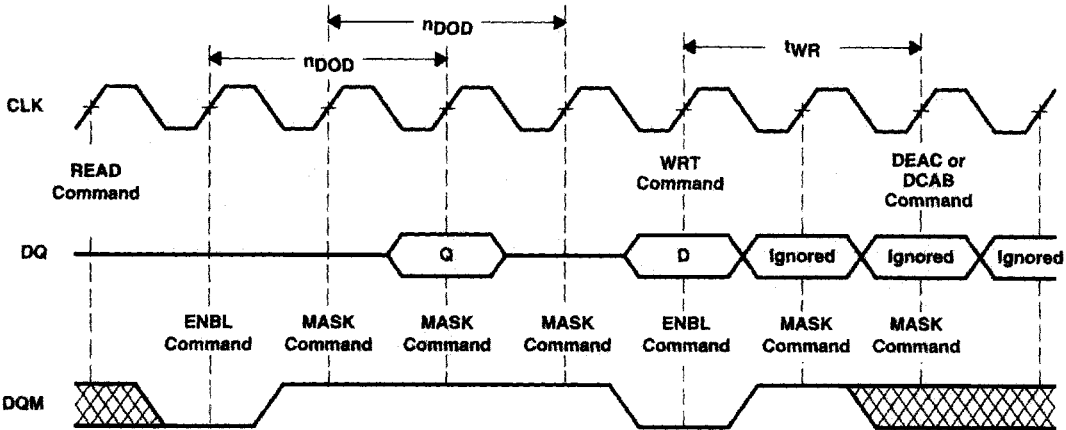
Figure 16. DQ Masking
