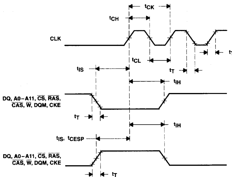
Figure 9. Input-Attribute Parameters
