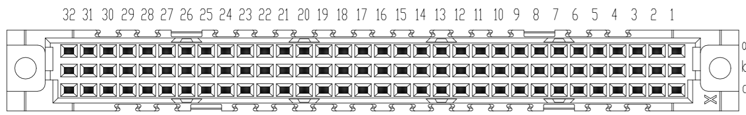
Leiterplatten-Lochbild / PCB drillhole Pattern
