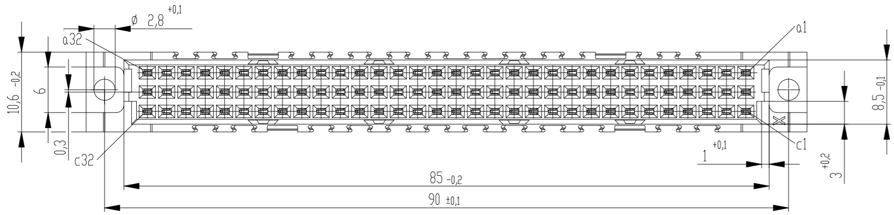
Bestückungsplan / contact layout
