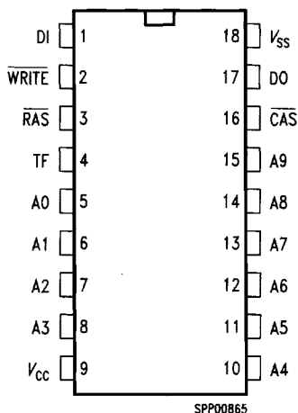
P-DIP-18-2
