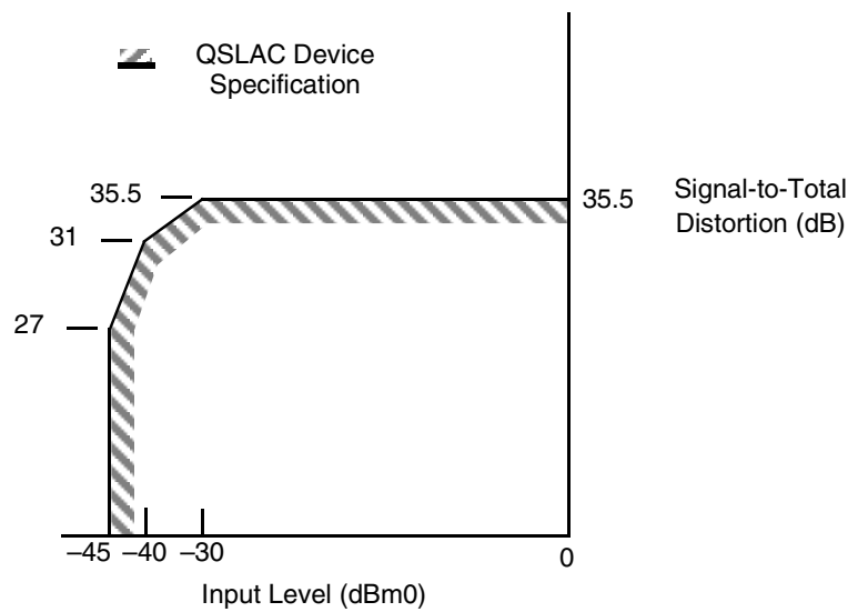
b. μ-law
