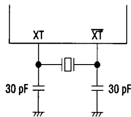
Figure 16.2 CSA4.09MGU
